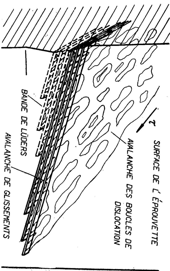
Fig. 1. Bande de Lüders (les hachures indiquent que la partie de la bande de Lüders se forme par les dislocations qui se déplacent lentement et les traits indiquent l'avalanche des glissements).
